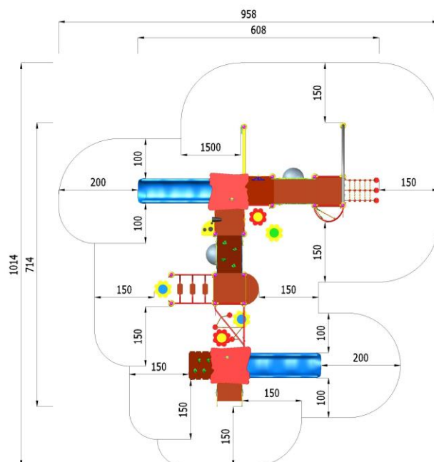
Безопасна зона на падане – 70.77 кв. м.:
